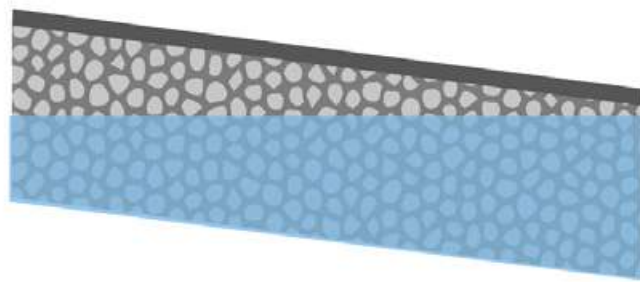
Compartiment de chaussée à structure réservoir
