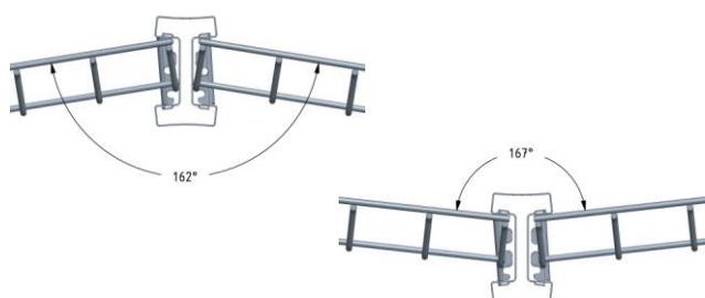
Assemblage avec panneau petit pli sans découpe
