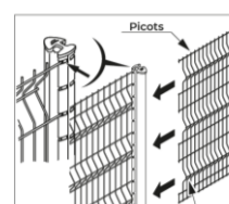
5 Engager le deuxième panneau. Renouveler les opérations. À la fin du chantier, retirer les bloqueurs universels (réutilisables).
