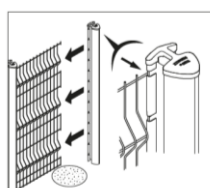
3 Engager le deuxième poteau sur le panneau.
