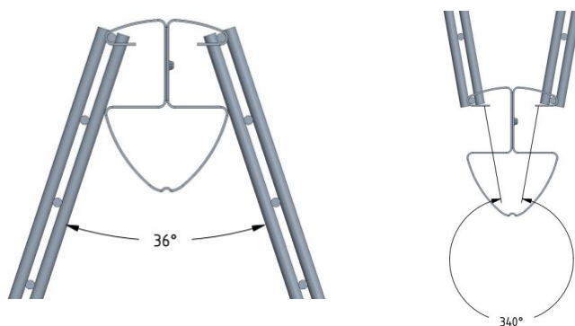
Assemblage avec panneau plat
