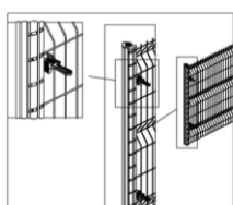
2 Positionner 2 bloqueurs universels pour maintenir en position le panneau sur le poteau, le temps du durcissement des scellements.
