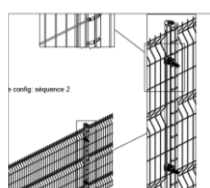
4 Positionner 2 bloqueurs universels et sceller le deuxième poteau.
