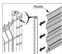
1 Sceller le premier poteau et engager le premier panneau (picots orientés en haut ou bas).
