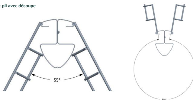
Assemblage avec panneau petit pli avec découpe
